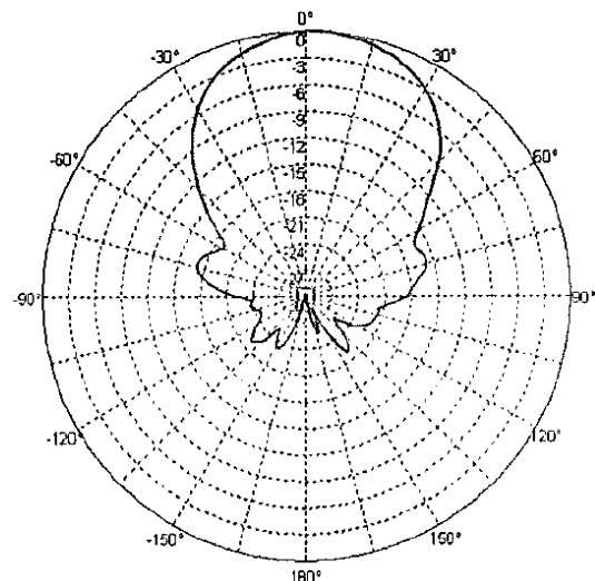
5 GHz
