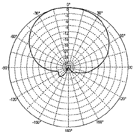
2.4 GHz
