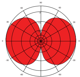
E-plane: 136 MHz
