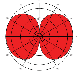
E-plane: 400 MHz
