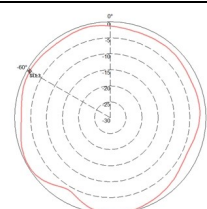
H-Plane Pattern
